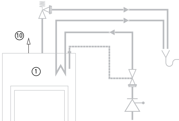
Abb. 3.4 Einbau der selbsttätigen Schnellentlüfter
