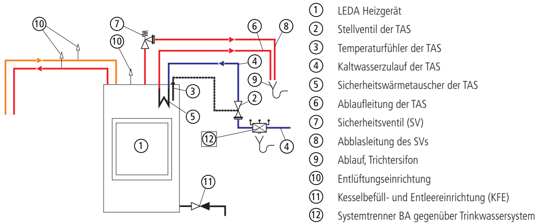
Abb. 4.1 Sicherheitseinrichtungen, Übersicht
