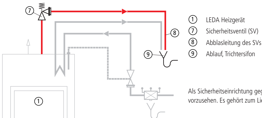
Abb. 4.2 Einbau des Sicherheitsventils
