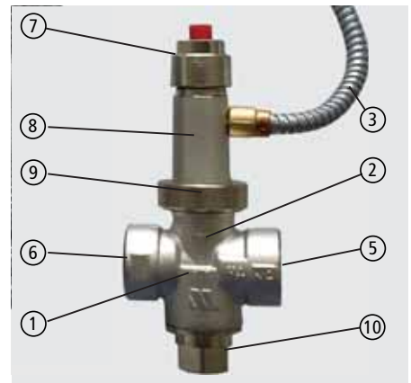
Abb. 7.5 TAS-Stellventil, Bauteile
