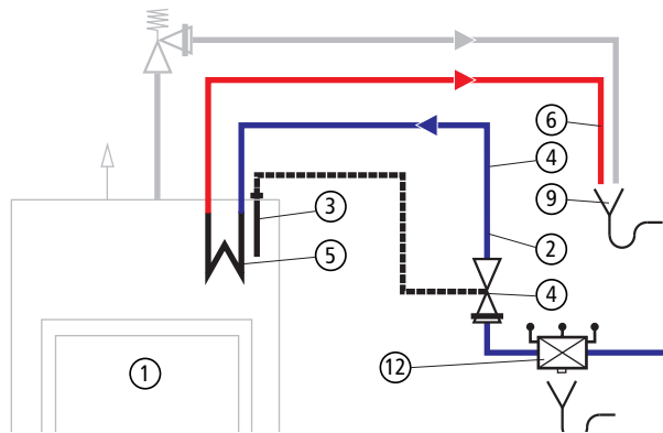
Abb. 4.3 Einbau der thermischen Ablaufsicherung (TAS)
