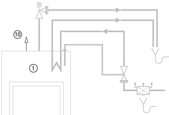
Abb. 4.4 Einbau der selbsttätigen Schnellentlüfters
